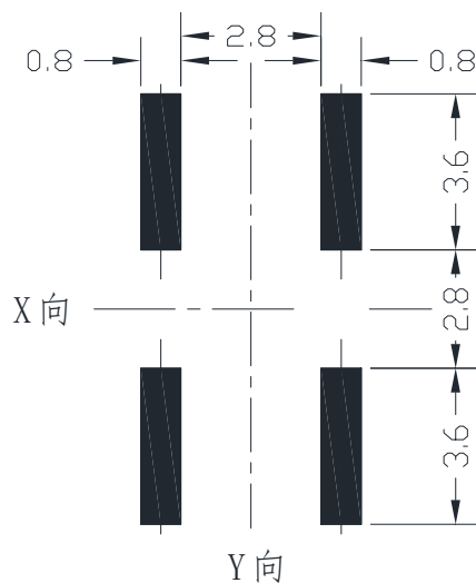
推荐焊盘尺寸图
