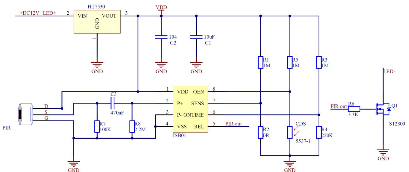
模拟 PIR+数字芯片 (ISB01) 应用参考图
