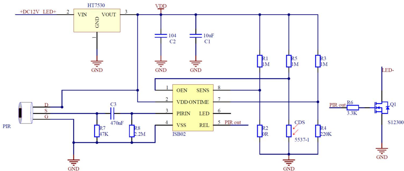
模拟 PIR+数字芯片 (ISB02) 应用参考图
